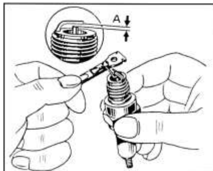
Рис. 9.9. Проверка зазора между электродами свечи
