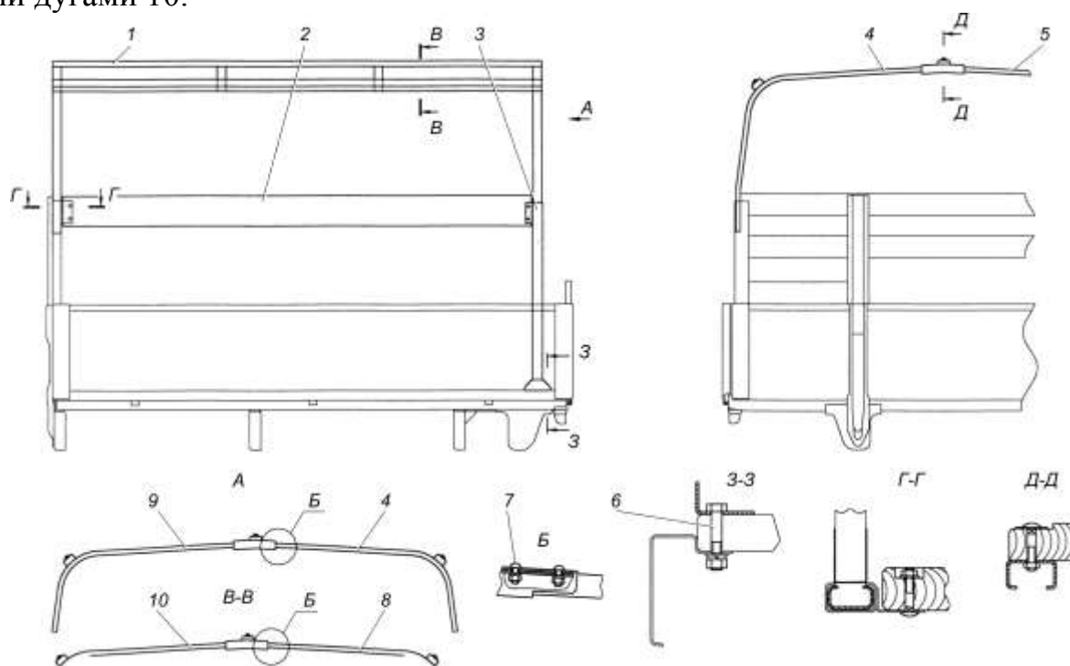
Рис. 12.3. Установка деталей каркаса тента:
