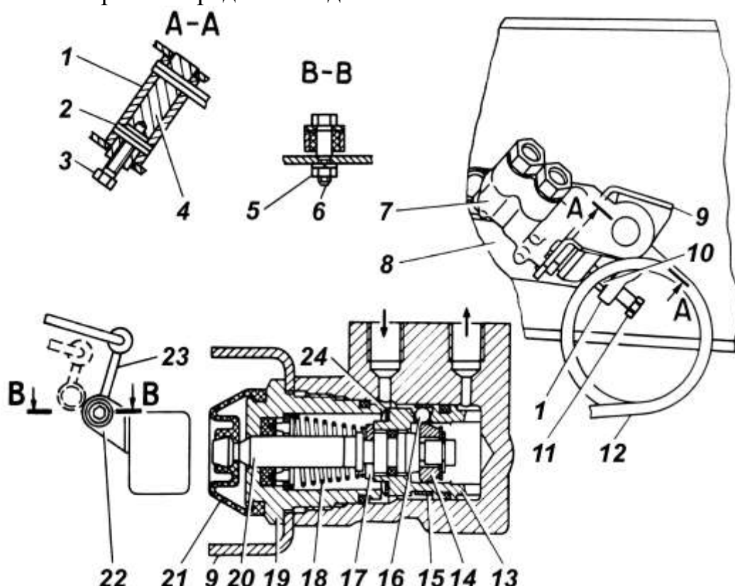
Рис. 9.8. Регулятор давления:
